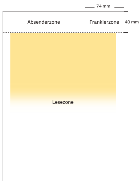
Abb. 24a – Hochformatige Sendung
